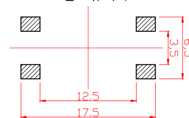
PCB. 焊接图
