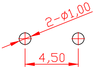
PCB. 焊接图
