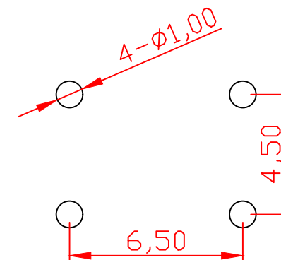
PCB. 焊接图
