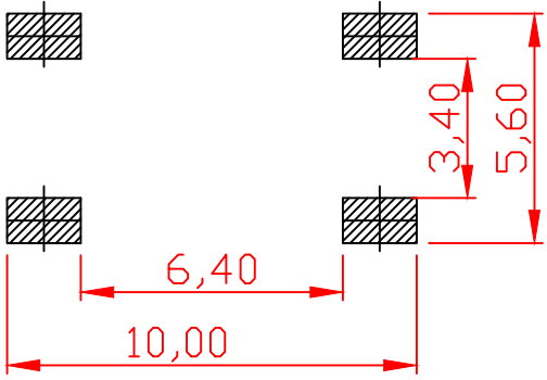
PCB. 焊接图
